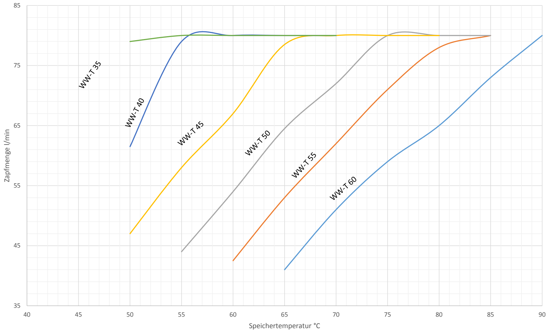
Auslegungsdiagramm 2er Kaskade
